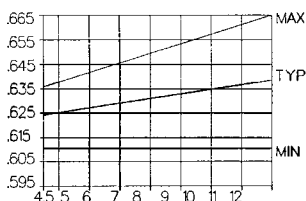
灵敏度 /V 与供电电压关系(mV/Gauss/V)
